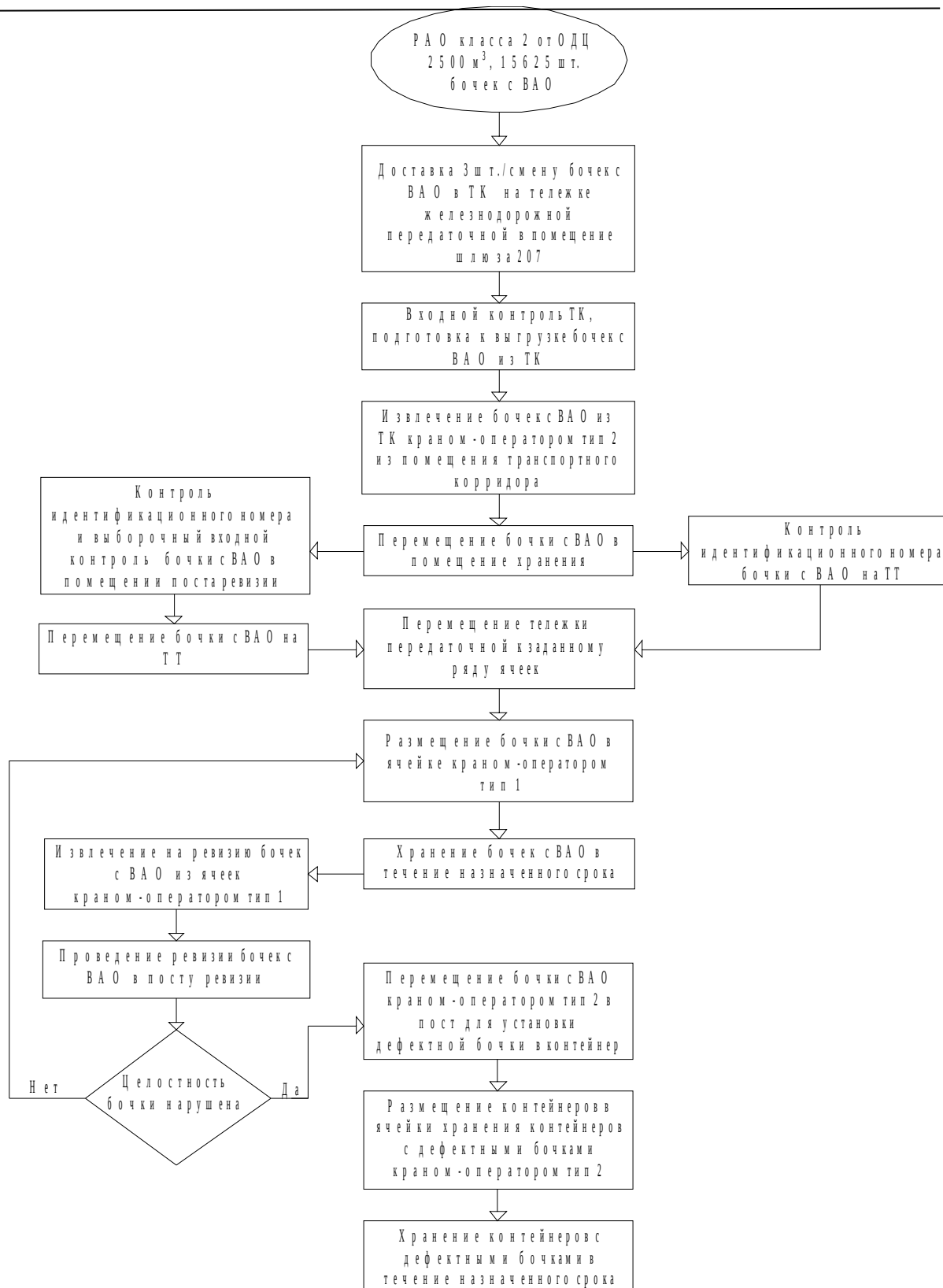
Рисунок 5.1. – Принципиальная схема обращения с бочками ВАО
